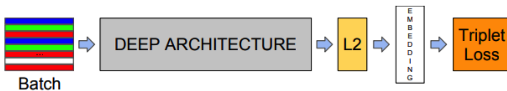
Hình 1.9. Kiến trúc của FaceNet [2]
