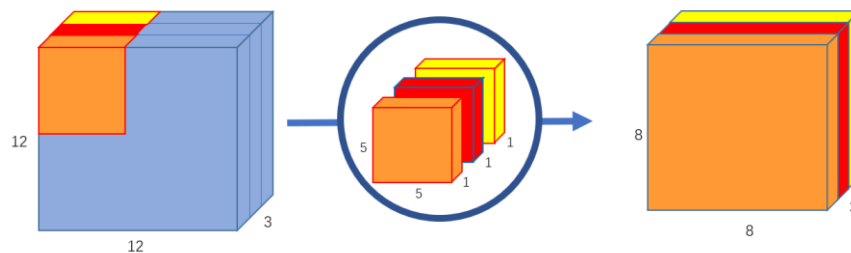
Hình 1.5. Cấu tạo depthwise convolution
