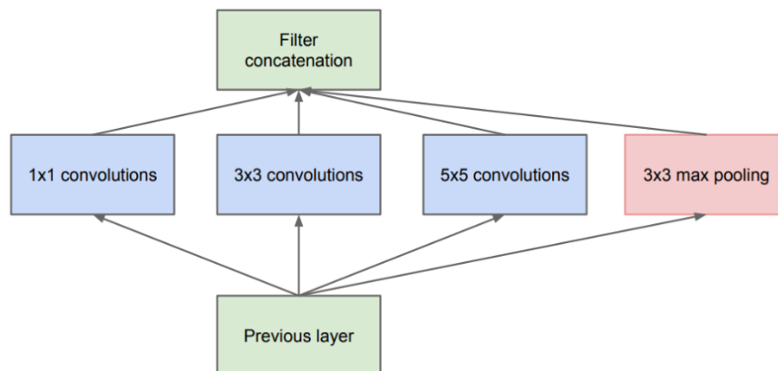
Hình 1.10. Inception module
