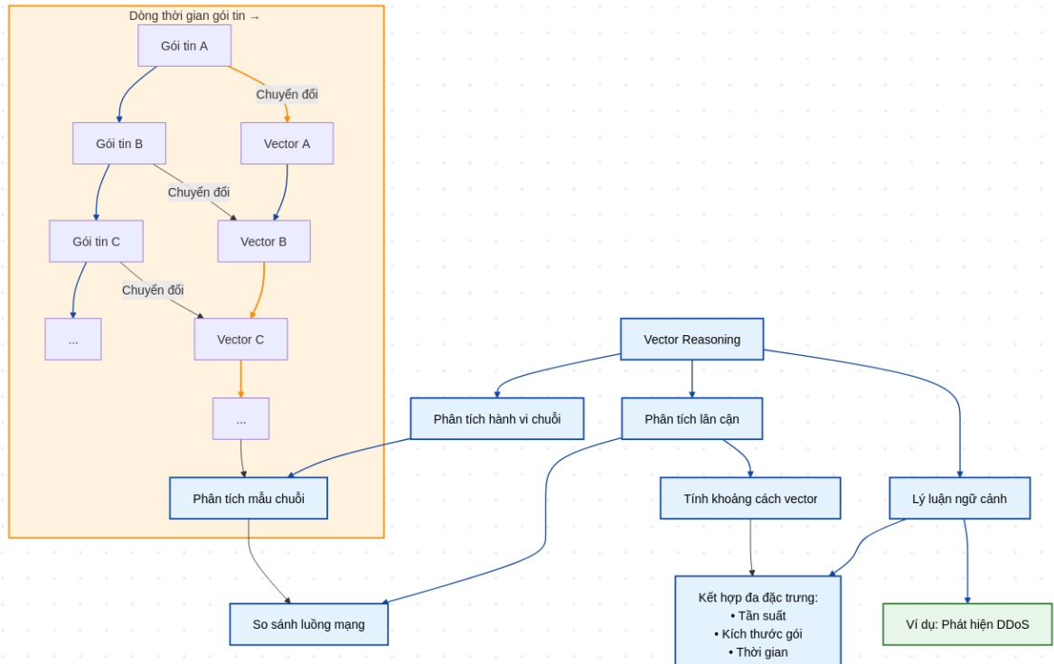
Hình 3.5: Phân tích, phát hiện DDoS
