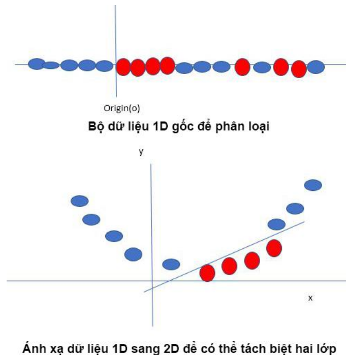
Hình 2.3: SVM sử dụng Kernel trong phân loại phi tuyến tính
