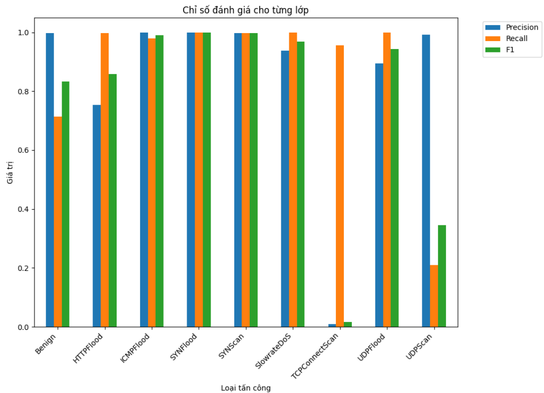
Hình 3.10: Các chỉ số kết quả Precision - Recall - F1
