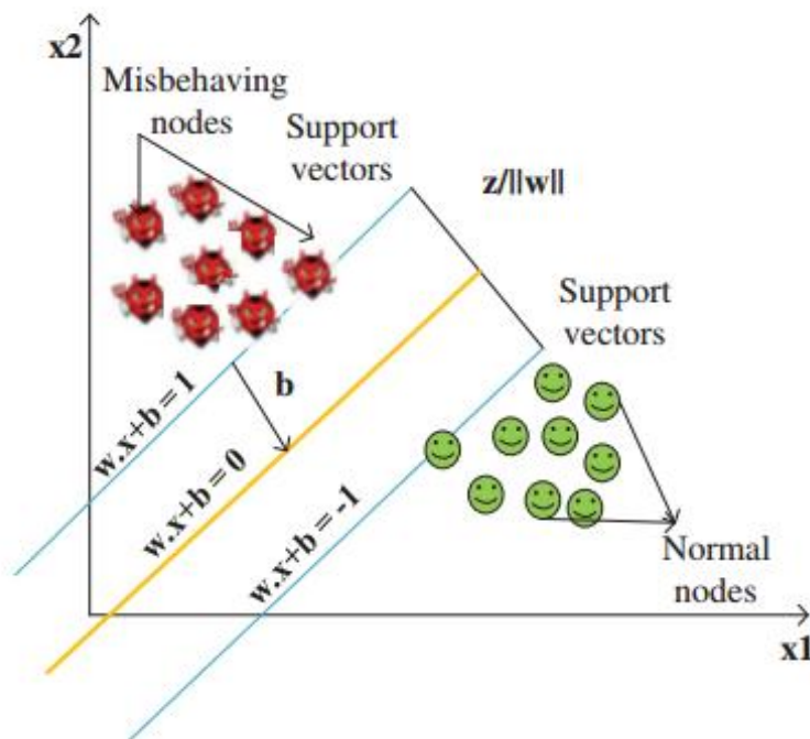
Hình 2.4: Phát hiện tấn công sử dụng SVM
