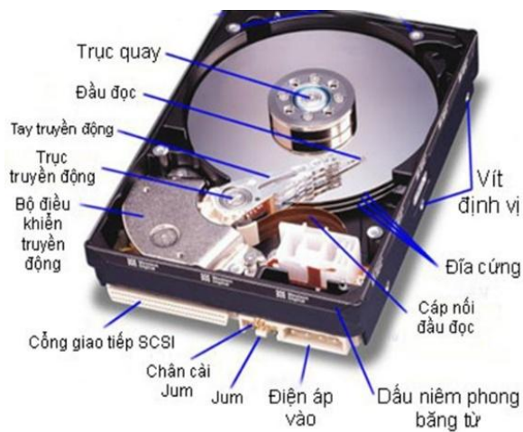
Hình 1.4. Cấu trúc ổ đĩa cứng Enterprise
