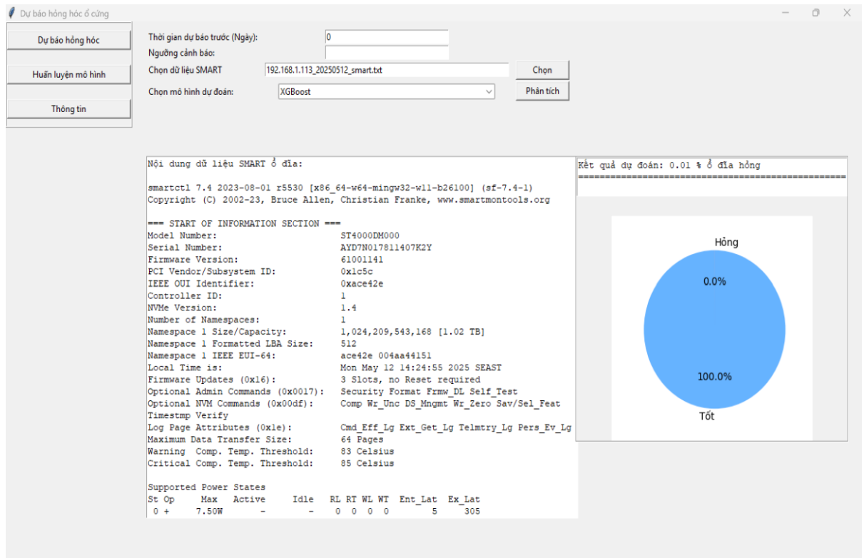
Hình 3.3. Kết quả dự báo hỏng hóc với dữ liệu thực tế với mô hình XGB
