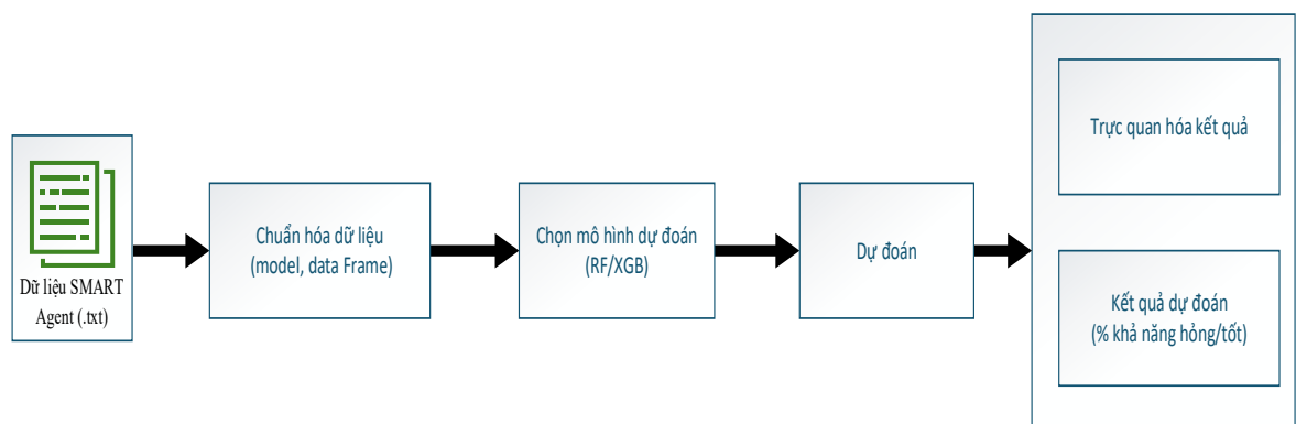
Hình 2.6. Tiến trình dự đoán phần trăm hỏng hóc ổ đĩa cứng
